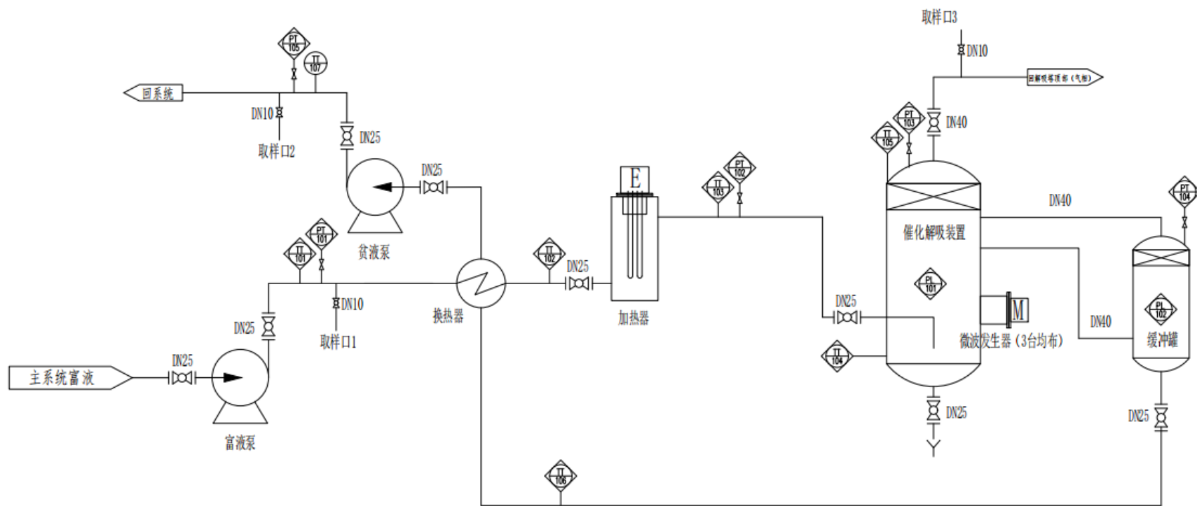
微波催化解吸试验装置流程图
