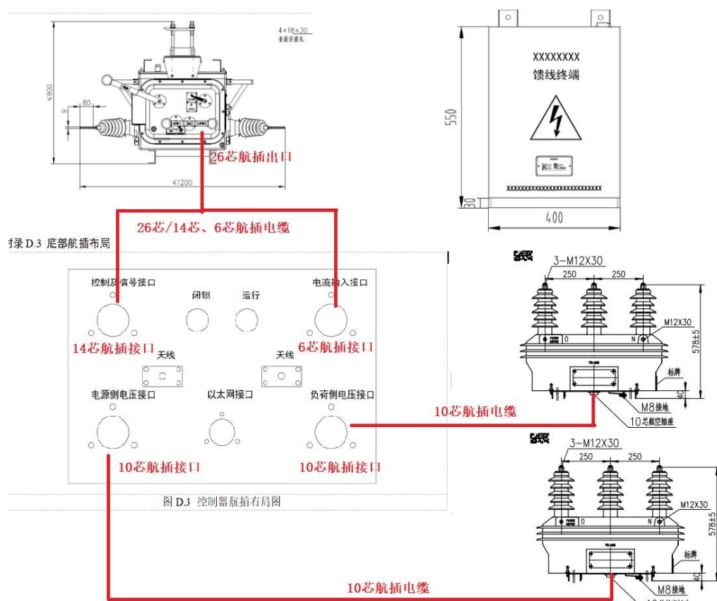
图 1 面向新型配电系统的即插即用保护装置接线图
